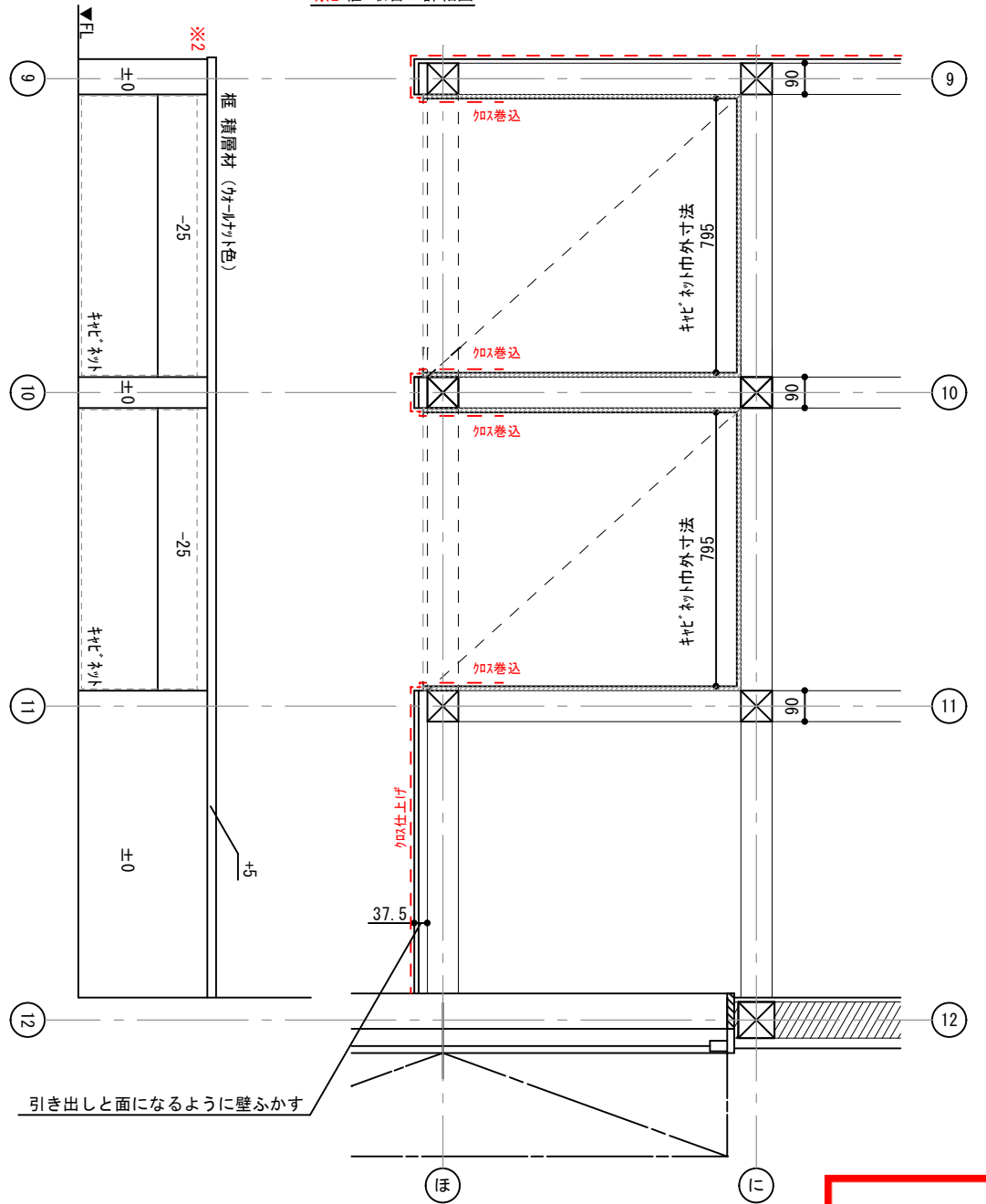
置コーナー 平面詳細図 1/20
