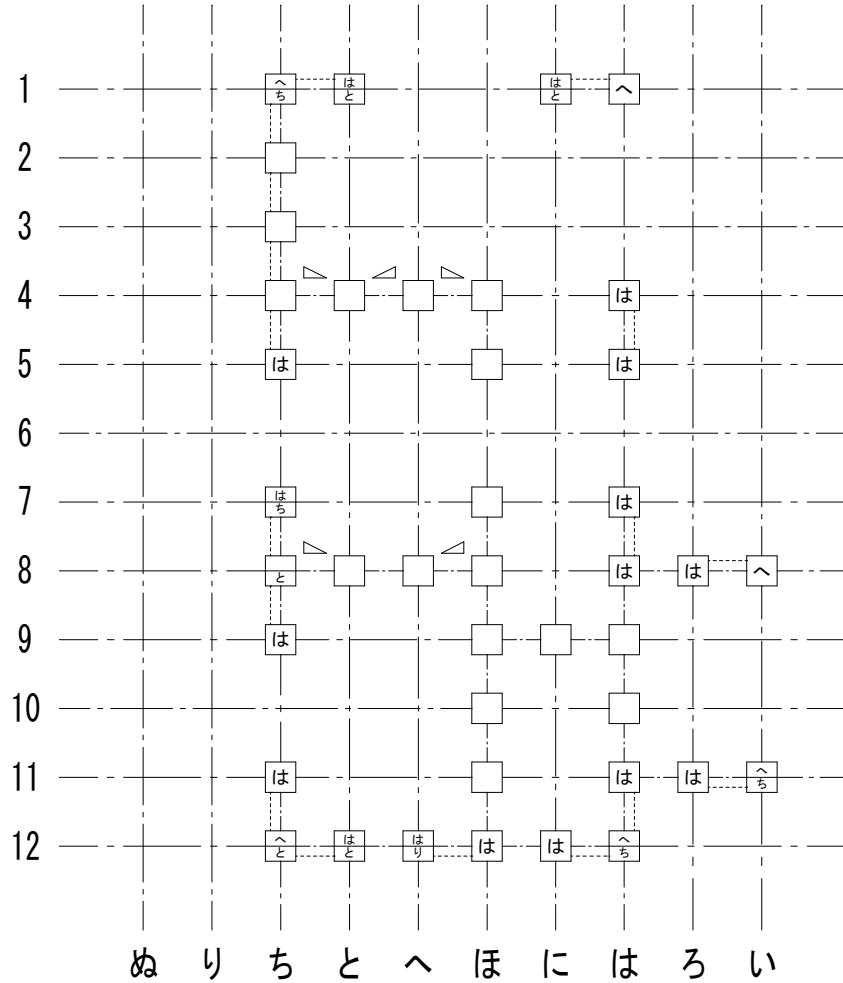
2 階柱壁伏図
