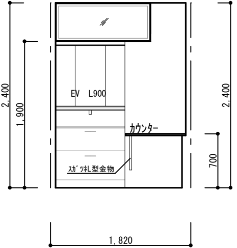
洗面所 北面
