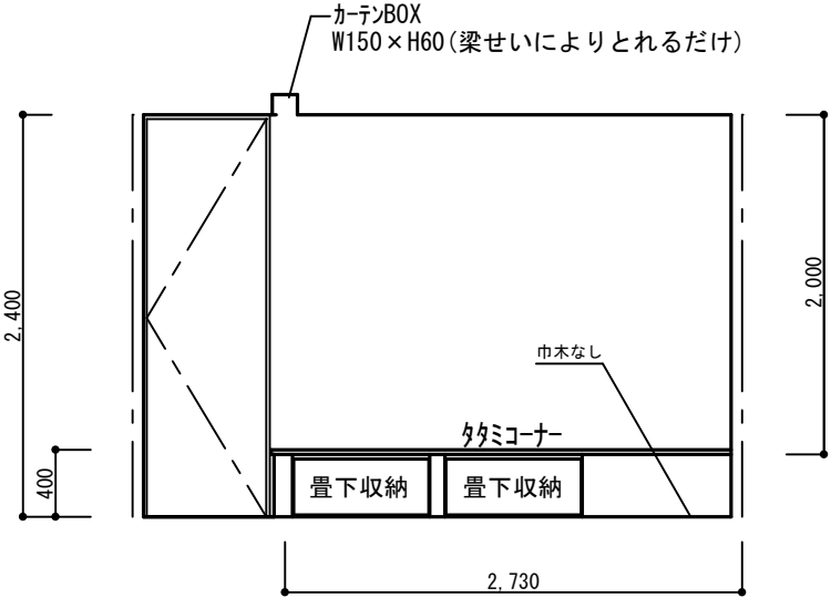
タタミコーナー 東面
