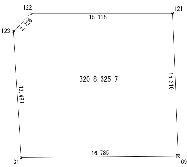
求積図 S=1 : 250
